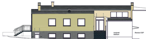
ELEWACJA POŁUDNIOWA 1:100
